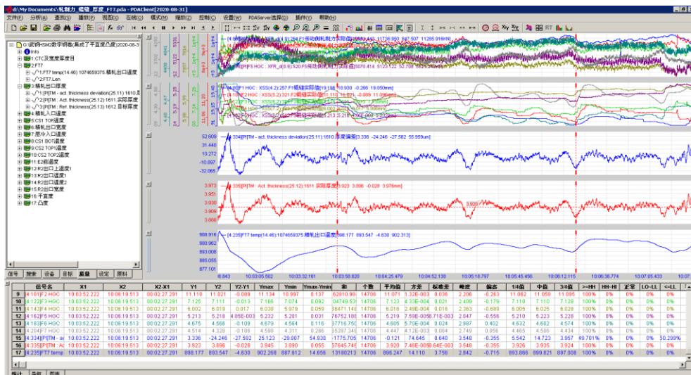
图 9.2 轧制力辊缝与出口厚度及 FT7 的关系
