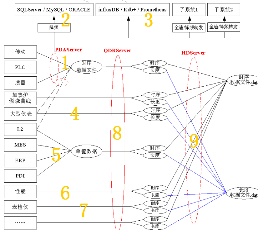
图 2.1 数字钢卷系统架构
