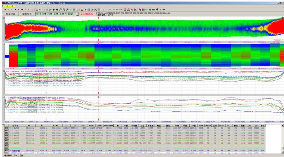
图 11.3 三维图形展示实测板形
