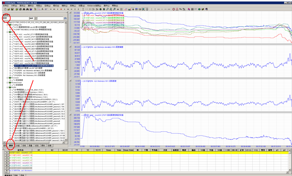
图 9.19 钢卷中的信号查找
