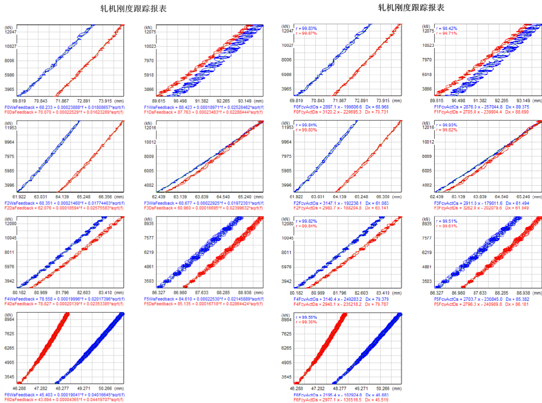
图 11.10 轧机刚度原始曲线和拟合曲线
