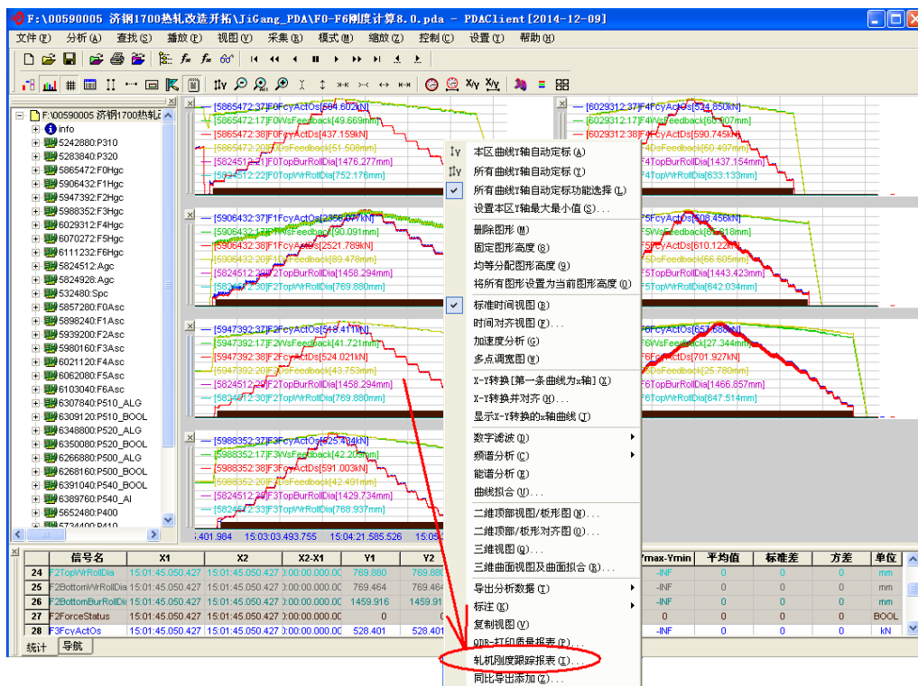
图 11.8 轧机刚度测量曲线
