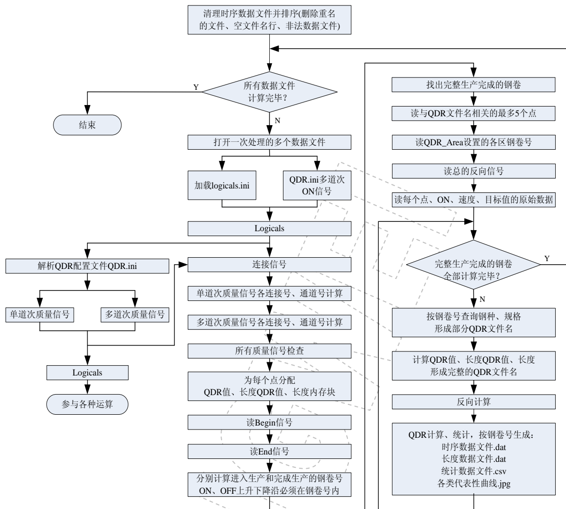
图 3.2 数字钢卷数据计算
