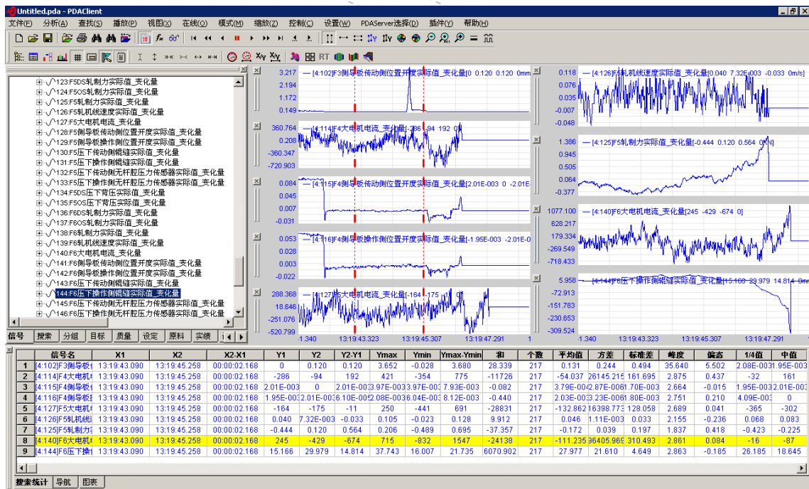
图 6.4 设备数字钢卷记录的曲线
