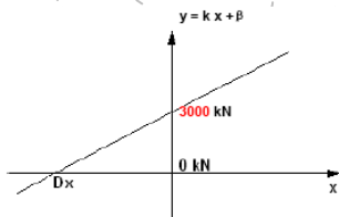
图 11.8 轧机刚度测量曲线
