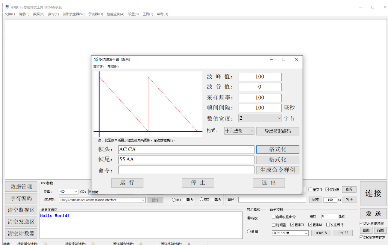
图 3-10-5 常用 USB 总线调试工具之反向锯齿波发生器
