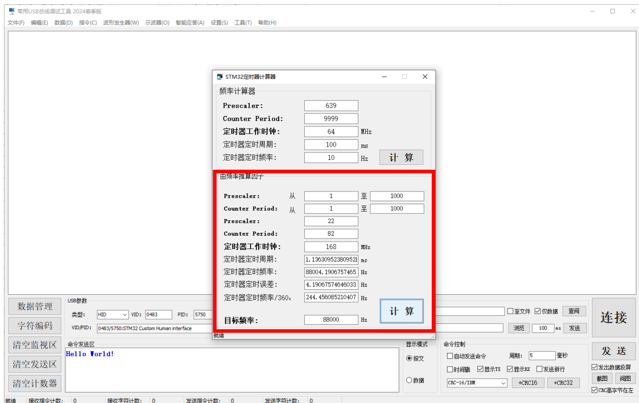
图 3-12-3 STM32 定时器计算器计算定时器频率
