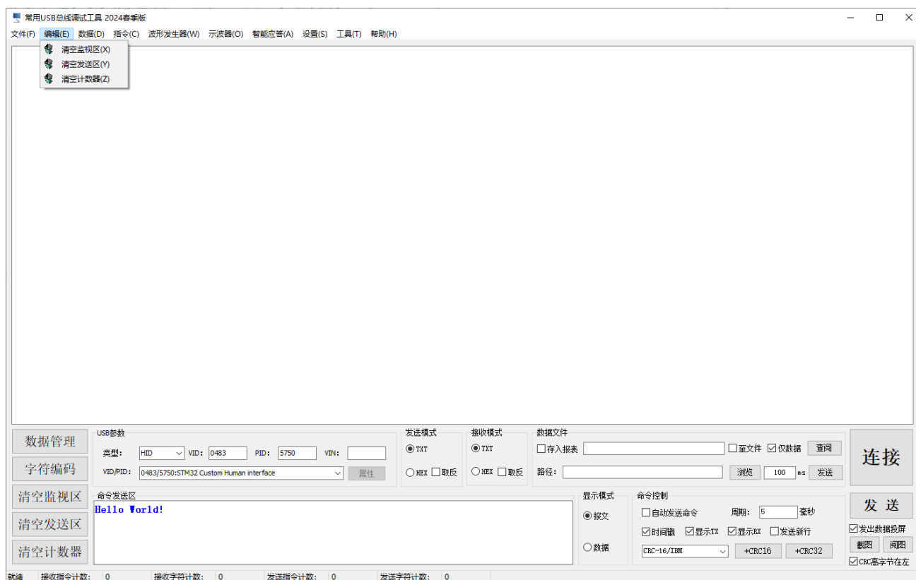
图 3-2 “编辑”菜单
