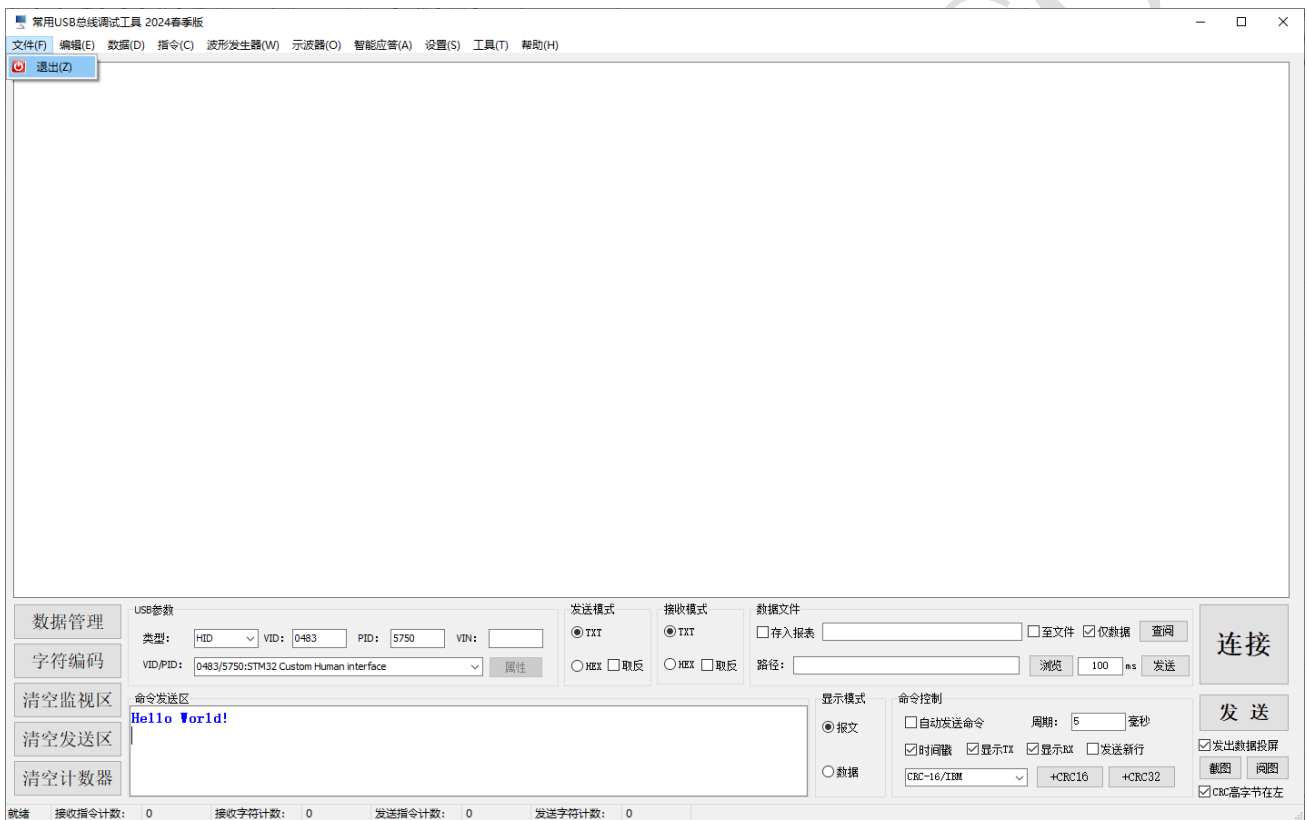
图 3-1-1 【文件】菜单
