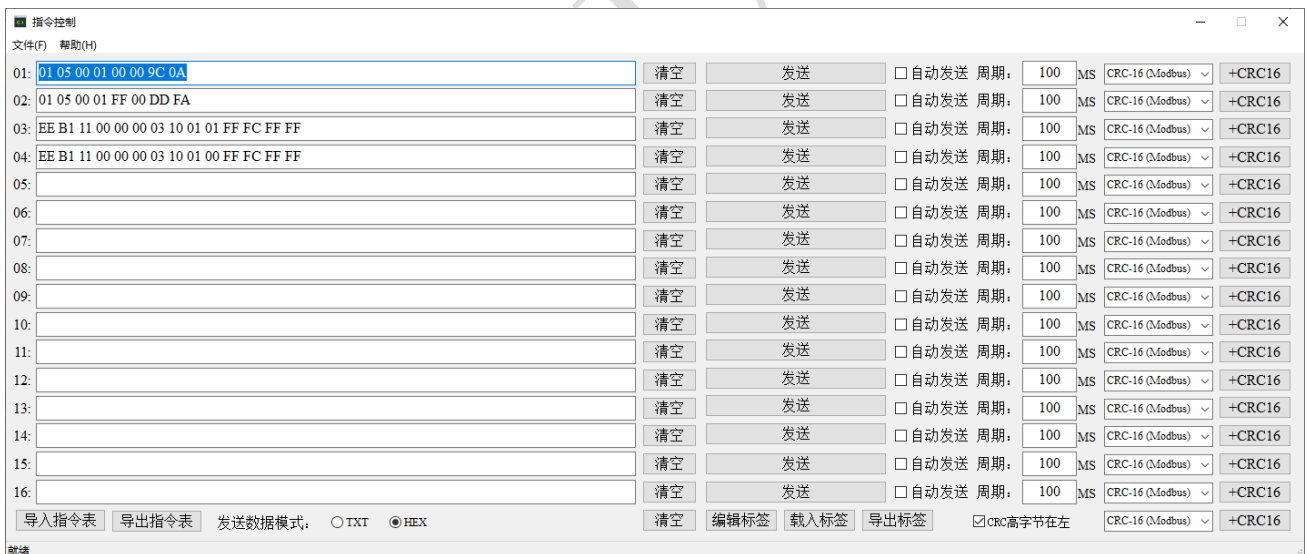
图 3-9-2 指令表窗体
