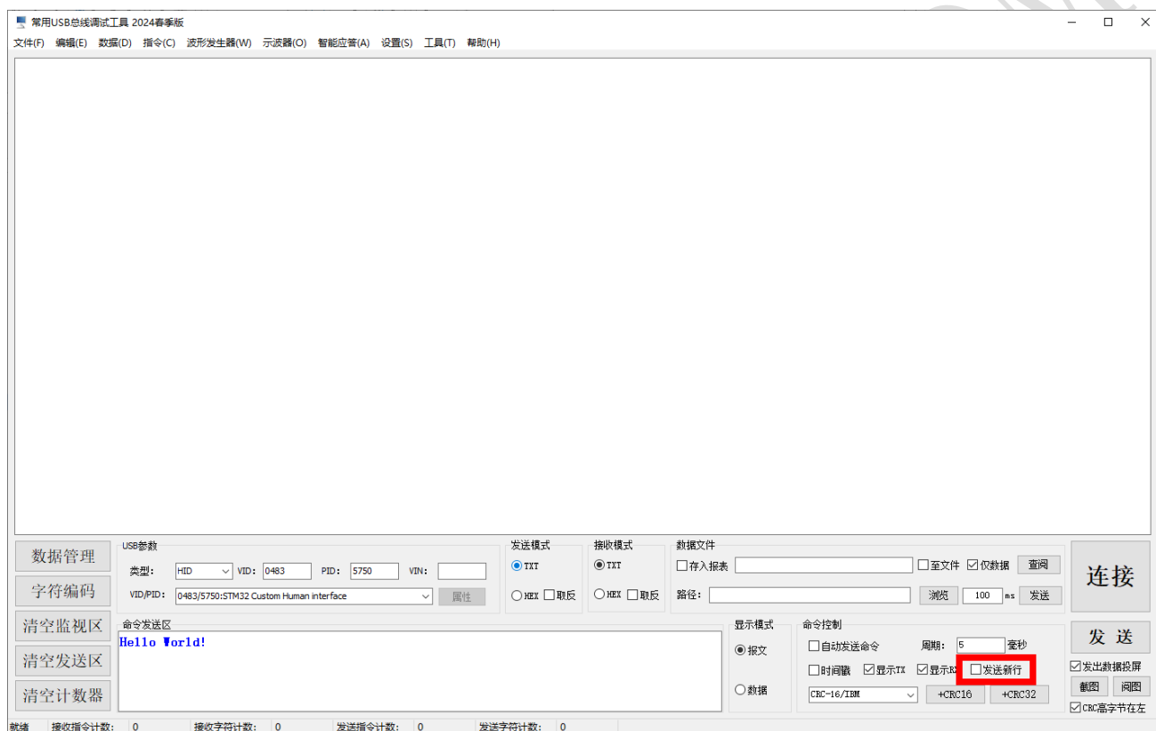
图 3-5 发送新行
