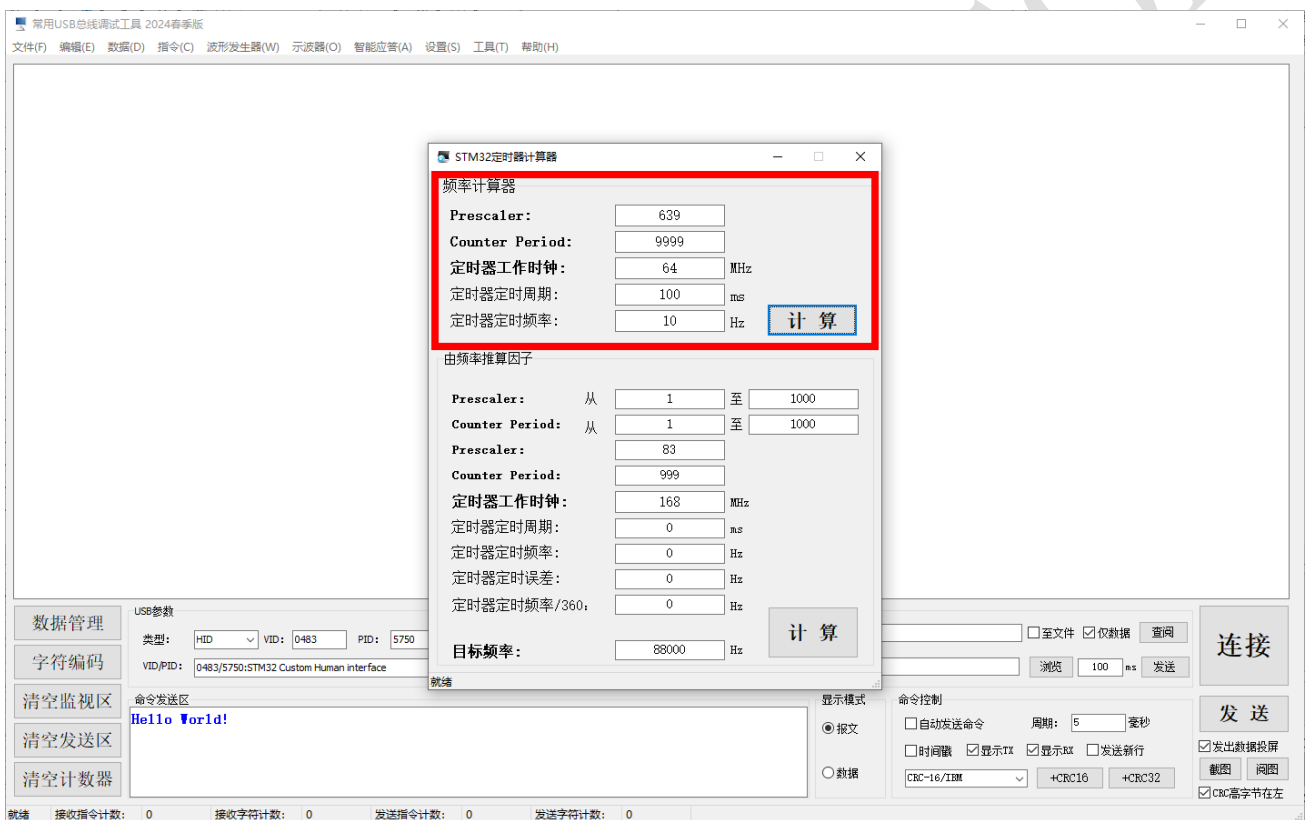
图 3-12-2 STM32 定时器计算器计算定时器频率
