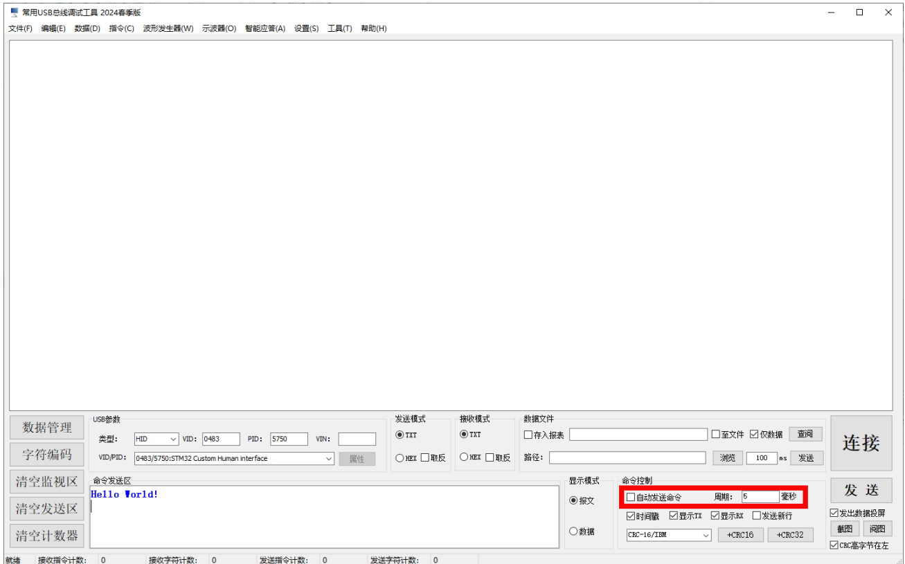
图 3-3 自动发送
