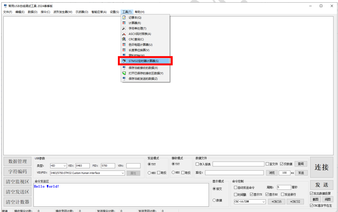
图 3-12 【工具】菜单
