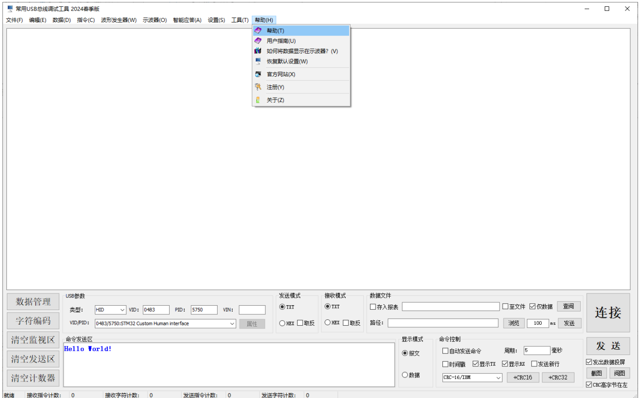
图 3-13 【帮助】菜单
